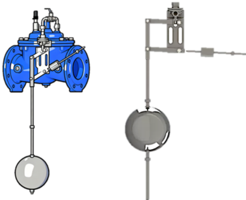
Float Valve 【Bi-lever】 ( /portal/article/index/id/176.html )
