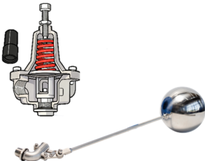
Float Valve 【Bi-lever】 ( /portal/article/index/id/176.html )
